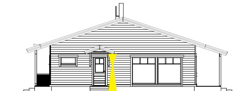
FASADI POHJOISEEN
