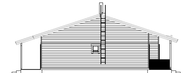
FASADI ETELÄÄN
